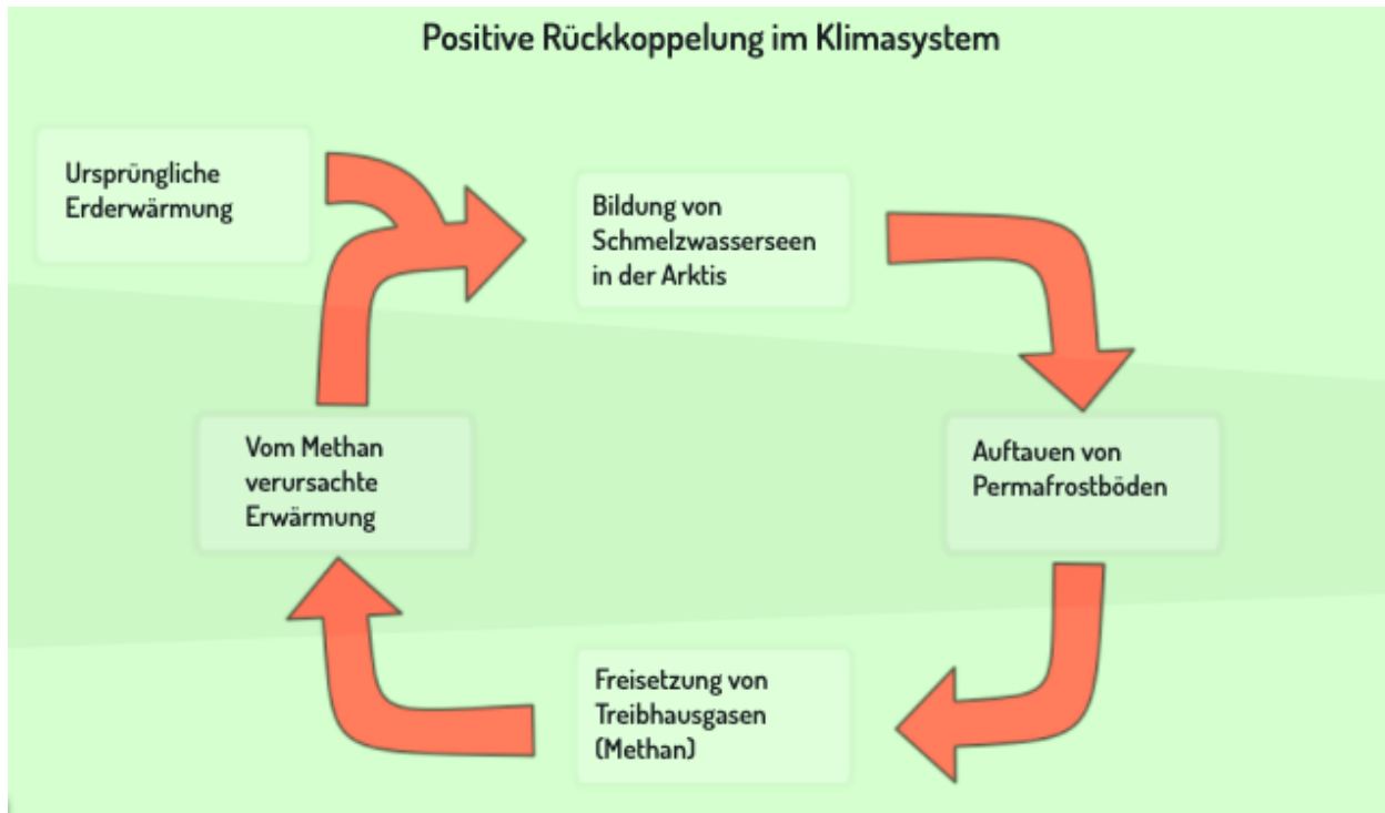
Abbildung 1: Die positiven Rückkoppelungen im Klimasystem.
